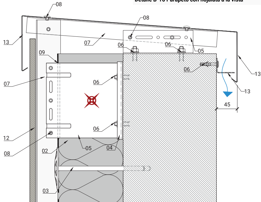
Detalle B-16 Parapeto con hojalata a la vista
