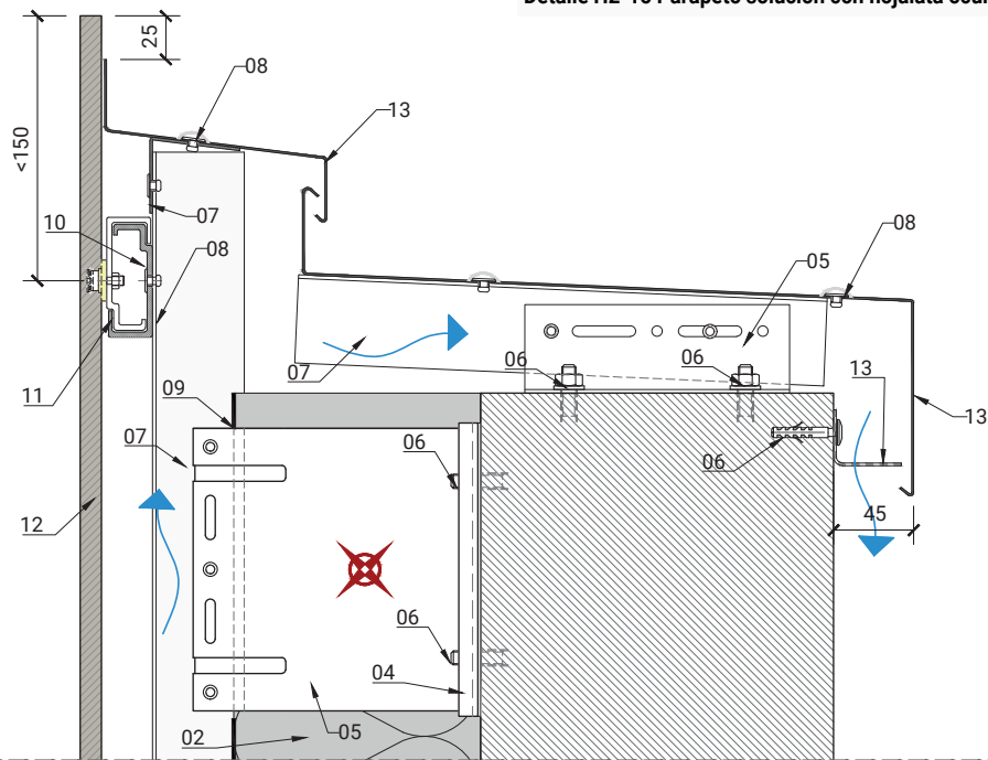
Detalle H2-16 Parapeto con hojalata a la vista
