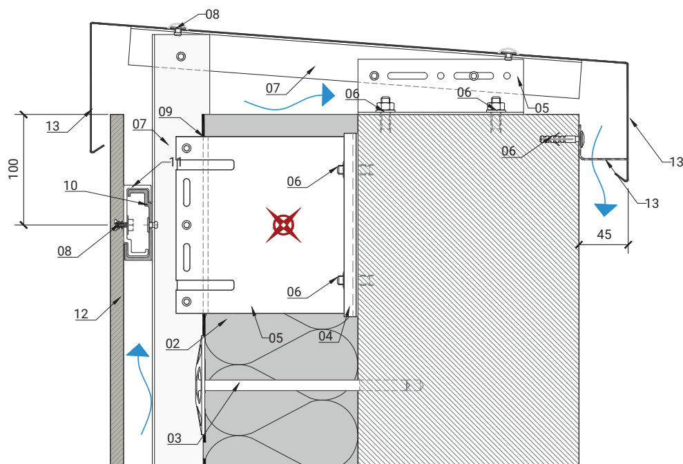
Detalle H1-16 Parapeto con hojalata a la vista
