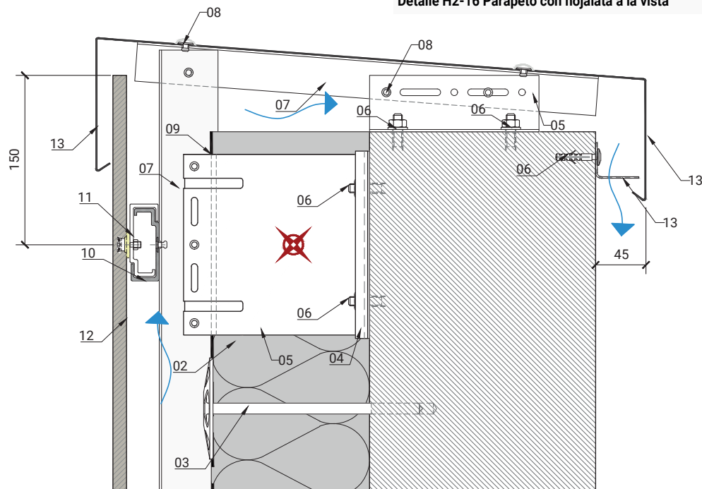
Detalle H2-16 Parapeto con hojalata a la vista
